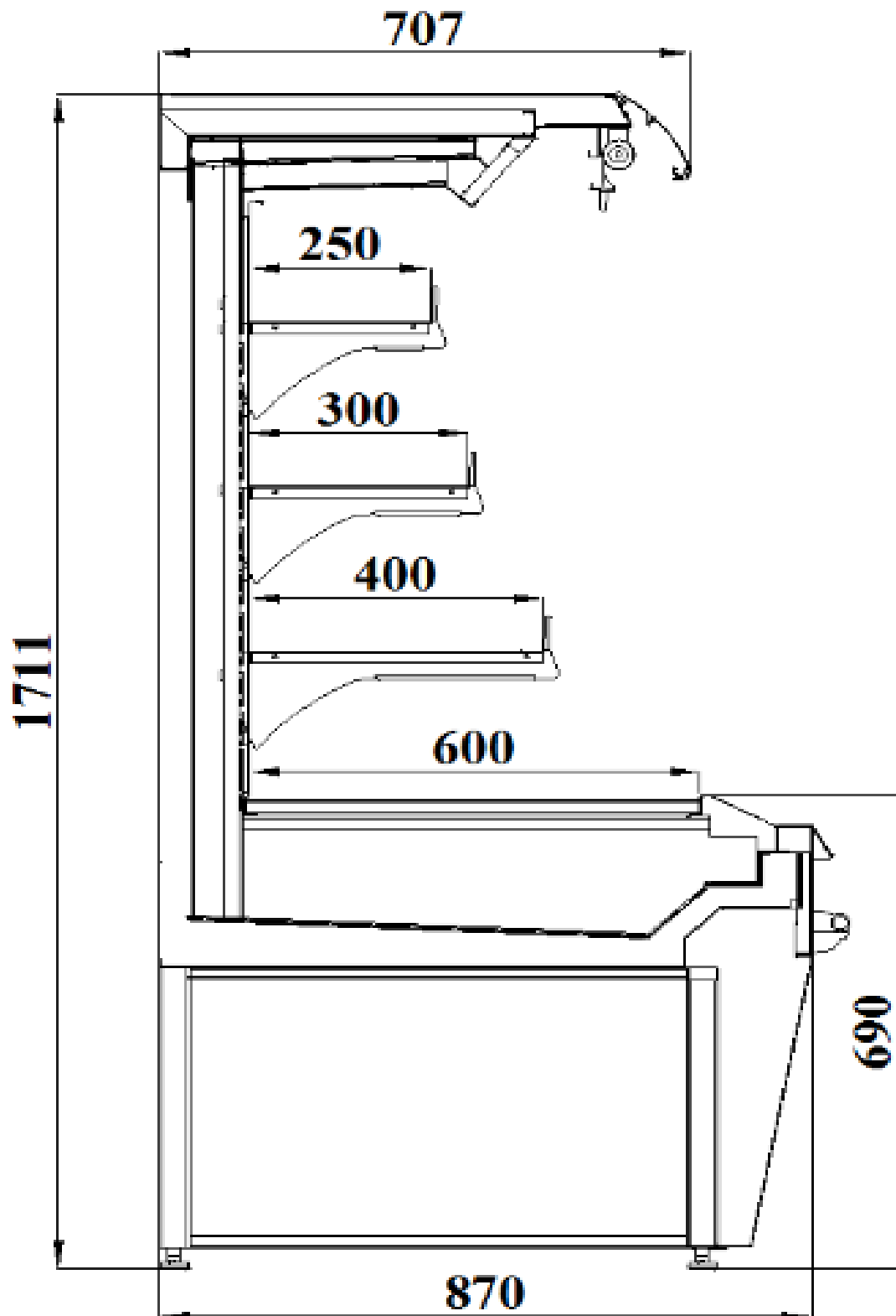
Querschnittzeichnung / Cross-sectional view
